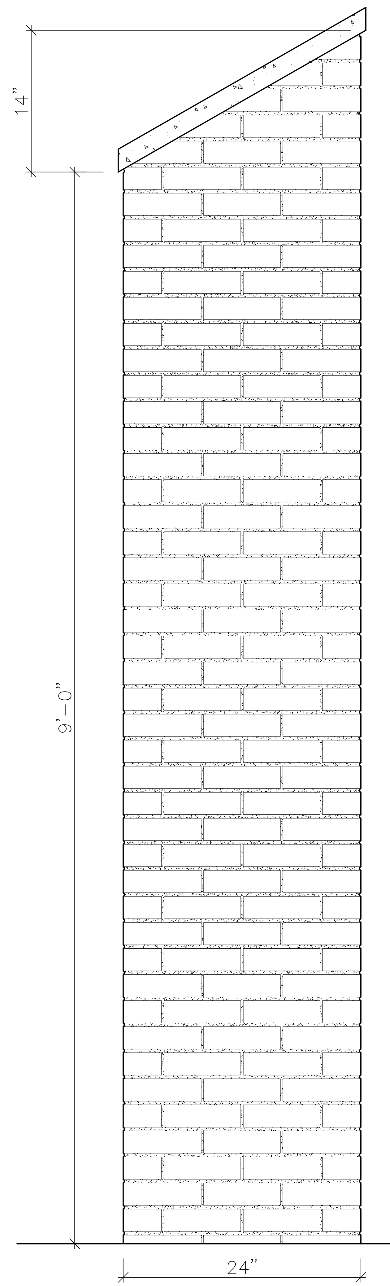
WALL END ELEVATION - HIGH END SCALE: 2" = 1'-0"
